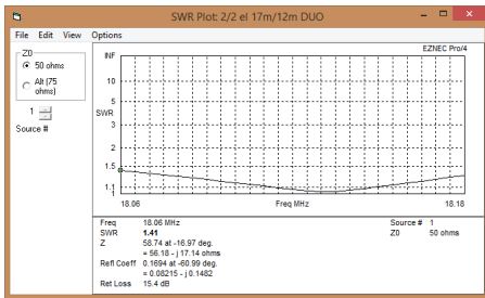
SWR 18MHz
