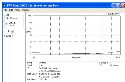
SWR 70MHz
